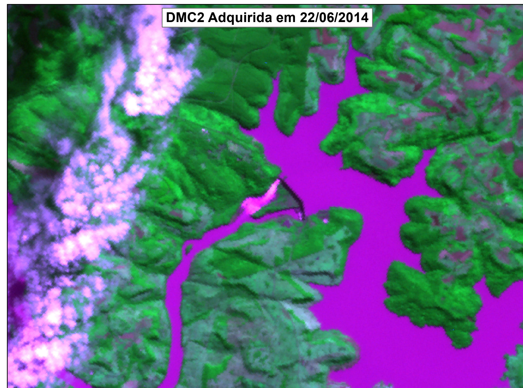
Barragem UHE Salto Osório
