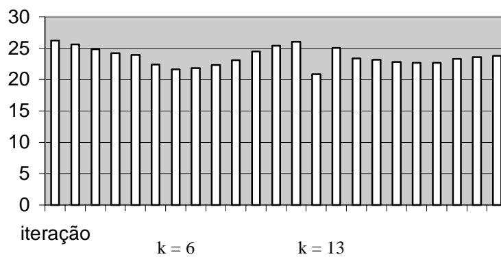
Figura 3: Valores de f ao longo da busca.
