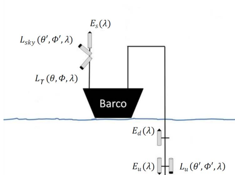
Figura 3.12. Configuração esquemática de sensores para medidas in situ de grandezas radiométricas recomendadas por protocolos de estudo da cor da água.
