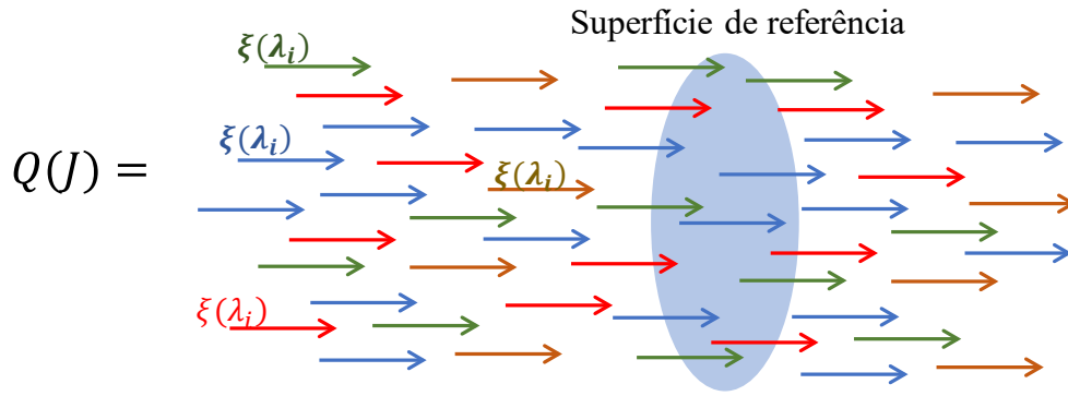
Figura 3.7. Campo de luz formado por fótons de diferentes comprimentos de onda ( \lambda ). Cada cor representa fótons de diferente quantidade de energia \xi(\lambda_i) . Setas azuis representam fótons da região espectral do azul, com maior energia. Setas vermelhas representam fótons da região espectral do vermelho, com menor energia. O círculo representa o referencial onde está sendo feita a medida. Esse círculo pode ser a superfície do detector de medida de energia radiante.
