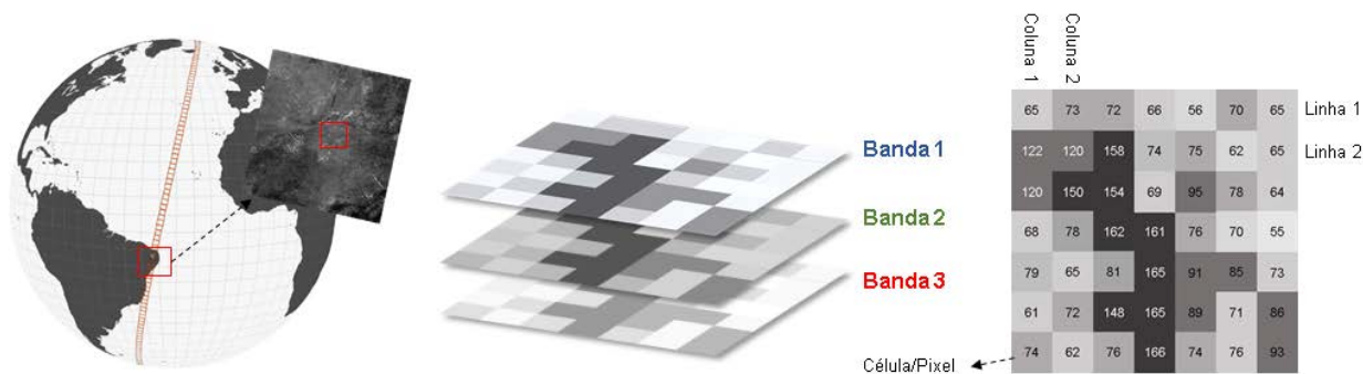
Figura 6.11. Modelo matricial da imagem.
