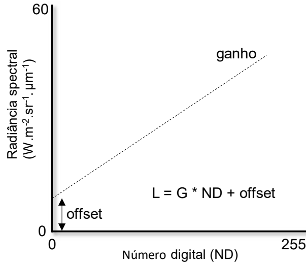
Figura 6.15. Calibração de imagens (ex.: 8-bits). O “ganho” (G) representa a inclinação da regressão linear, e o “offset” define a radiação espectral para ND igual a zero. A conversão de ND para radiação segue a equação linear ( L = G \times ND + \text{offset} ).
