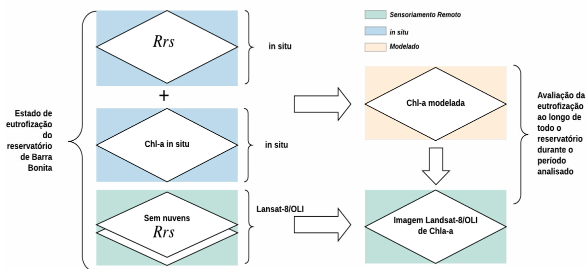
Figura 7.6. Fluxograma da metodologia adotada por Watanabe et al. (2015) para a estimativa da concentração de chl-a a partir de dados in situ e de imagens orbitais do sensor Landsat-8/OLI.
