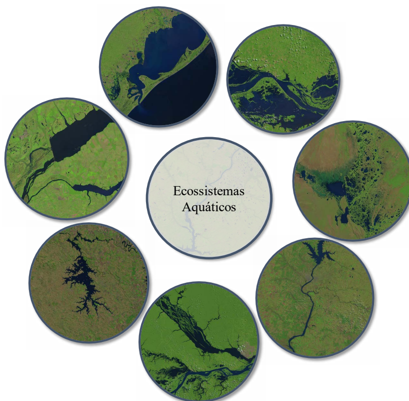
Figura 1.1. Sistemas aquáticos continentais: rios, lagos, represas, áreas alagadas, córregos etc.
