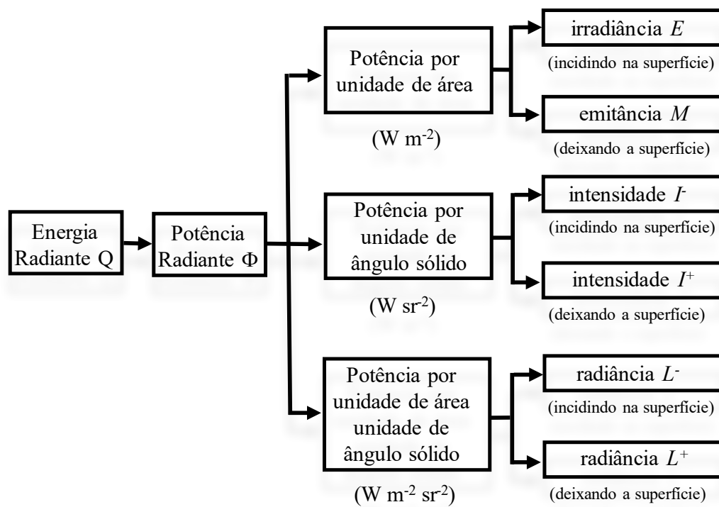
Figura 3.13. Hierarquia dos conceitos radiométricos. Adaptado de Mobley(1994).
