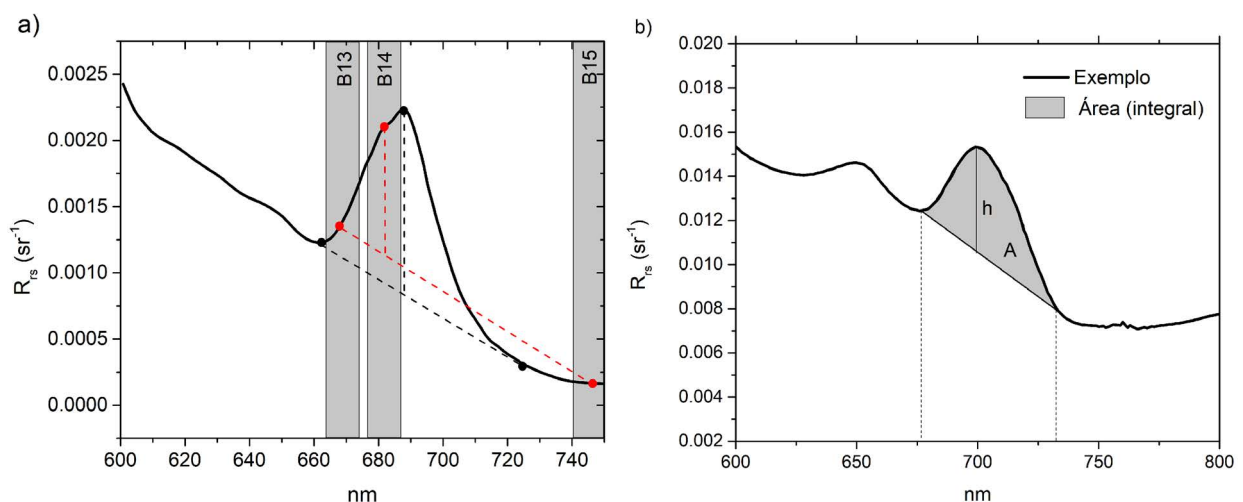
Figura 5.6. a) Exemplo de aplicação do método FLH para a determinação de fluorescência em águas costeiras usando bandas do sensor MODIS (Adaptado de Hoge et al., 2003). b) Determinação da altura (h) e área (A) do pico de espalhamento por células fitoplanctônicas.
