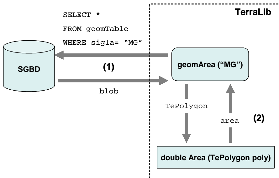
Figura 3.5 - Cálculo de área no TeDatabase
