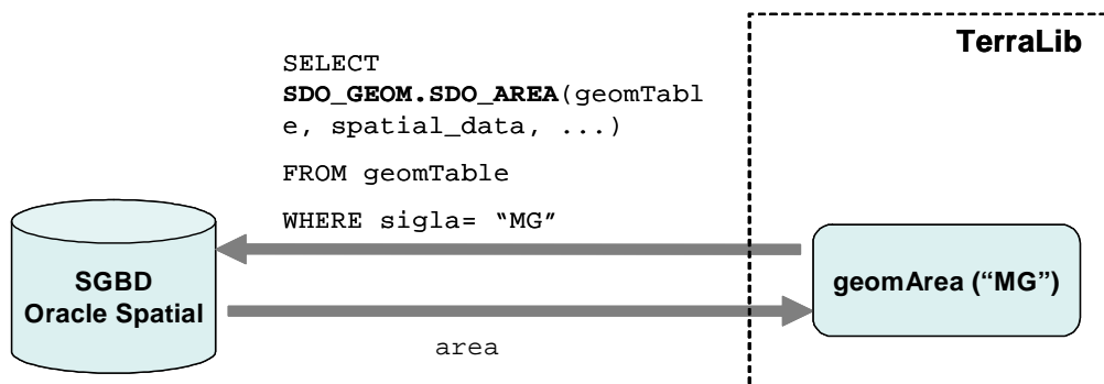
Figura 3.6 - Cálculo de área no TeOracleSpatial
