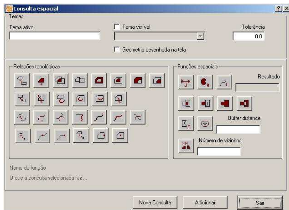
Figura 4.1 - Tela de operações espaciais sobre dados vetoriais
