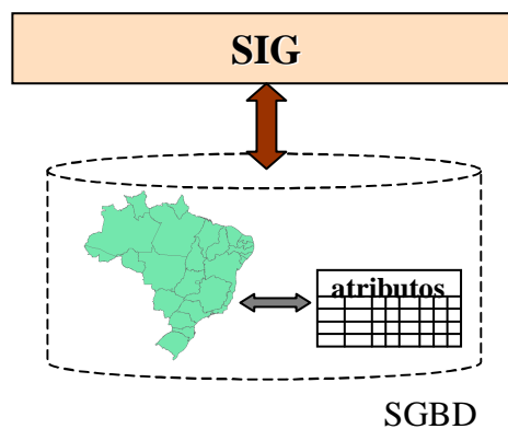
Figura 2.2 - Arquitetura Integrada
