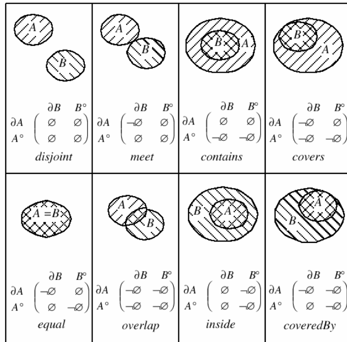
Figura 2.3 - Relações topológicas
