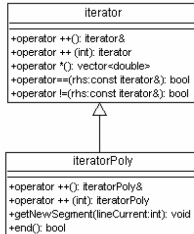
Figura 3.12 - Classe IteratorPoly
