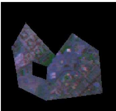
Figura 4.13 - layer Imagem_Brasilia_Mask_In
