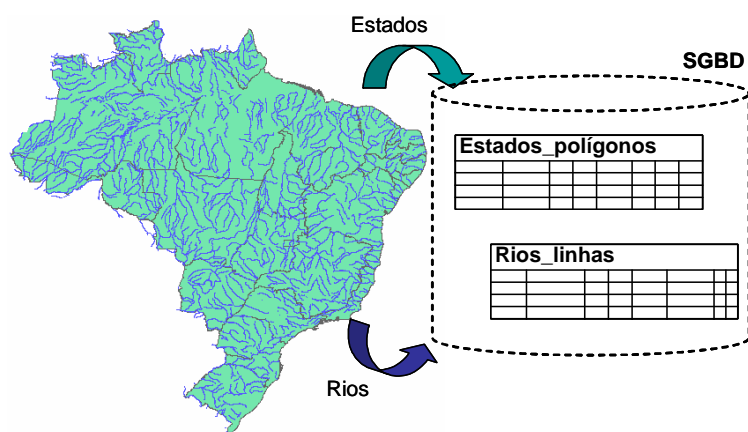
Figura 3.7 - Armazenamento de dados geográficos no SGBD
