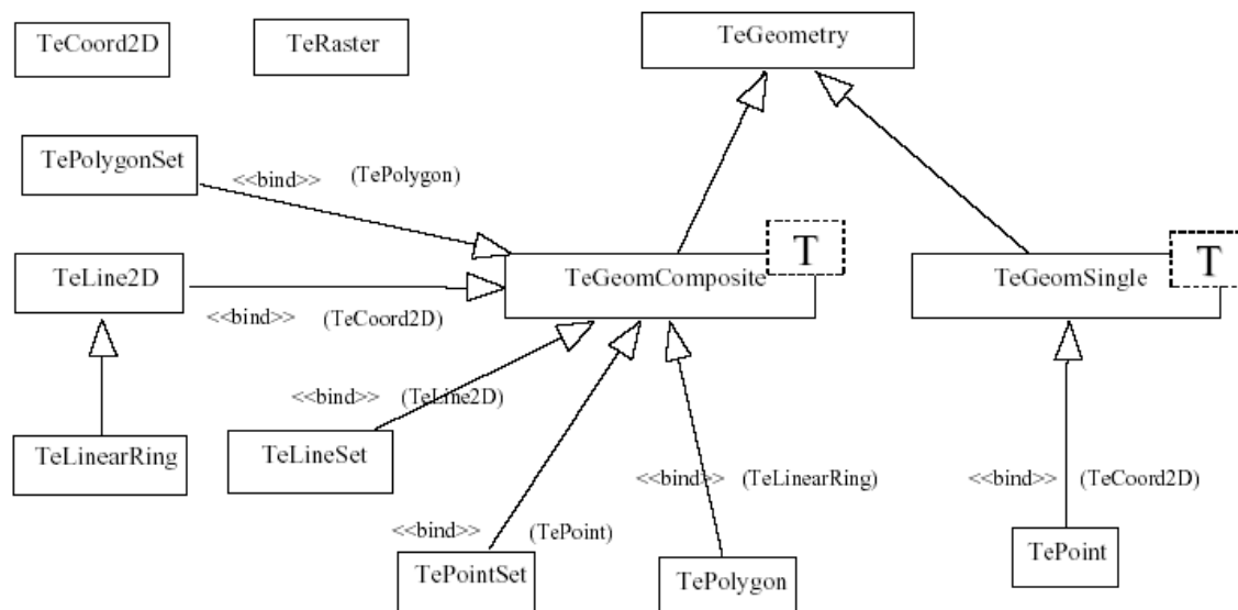
Figura 3.1 - Classes do Kernel da TerraLib
