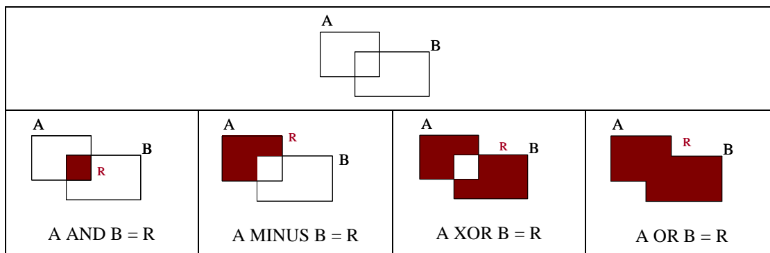
Figura 3.11 - Operações de conjunto
