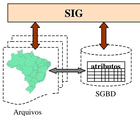
Figura 2.1- Arquitetura Dual
