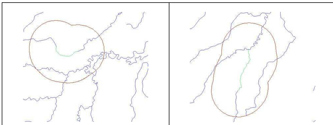
Figura 4.7 - Buffers gerados
