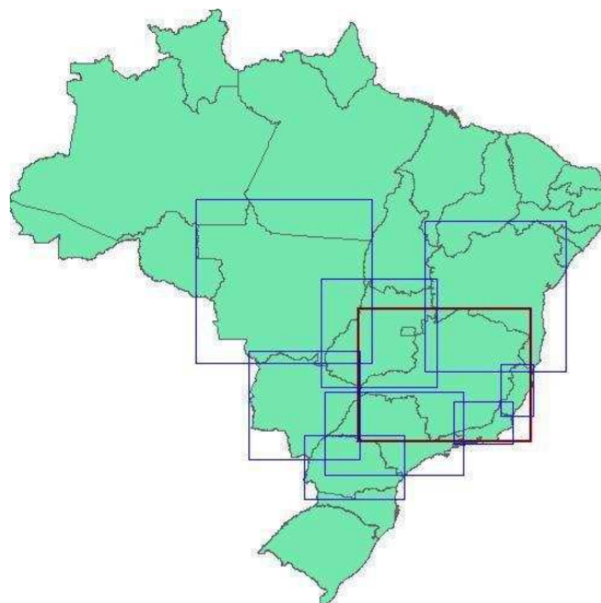
Figura 3.8 - Primeira etapa da consulta espacial
