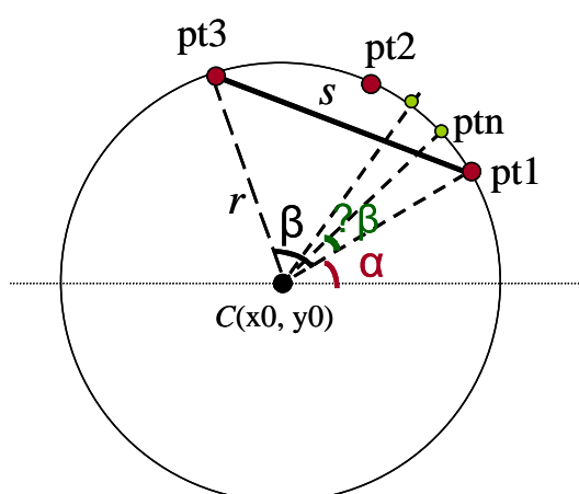
Figura 3.10 - Geração de um arco a partir de três pontos
